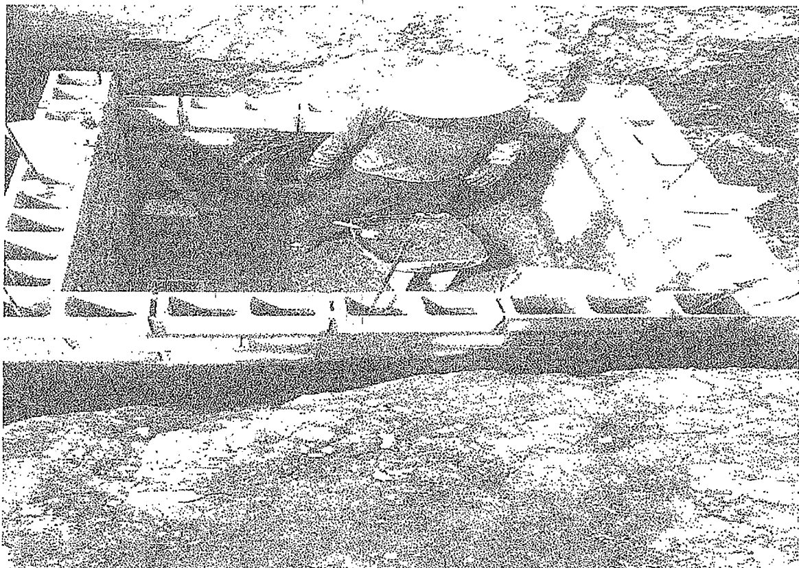
Execução do poço de visita da galeria de águas pluviais.
